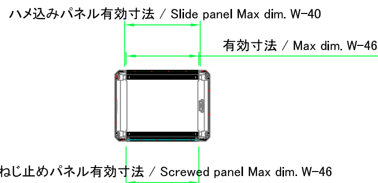
A-A ( 1 : 8 )
